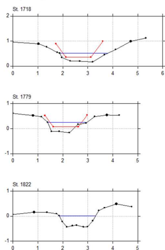
Figur 4: Tværprofil st. 1718 – 1822 meter af Fiskbæk Møllebæk sammenligning af opmåling fra 2021 og regulativet fra 1971
