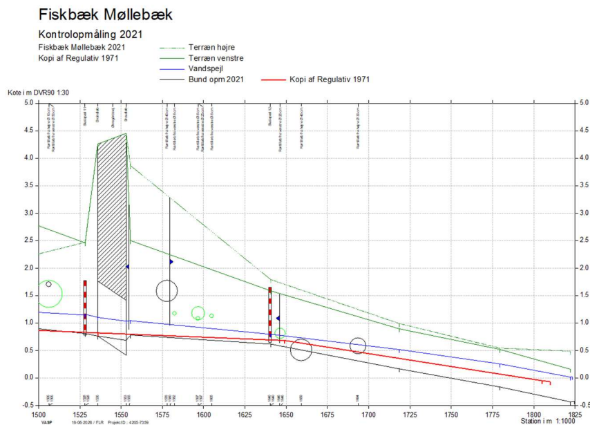
Figur 2: længdeprofil af Fiskbæk Møllebæk sammenligning af opmåling fra 2021 og regulativet fra 1971.
