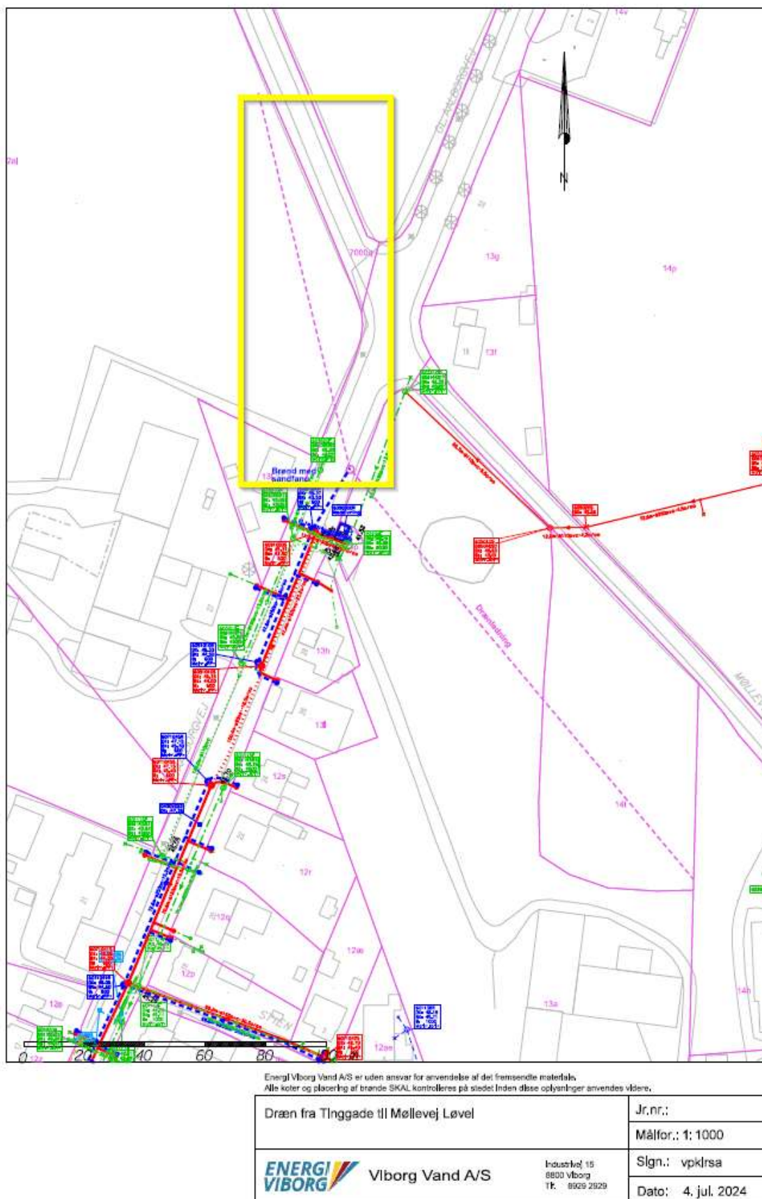
Figur 4. Gul firkant angiver dræn der skal udskiftes og bruges til overflade- og tagvand.
