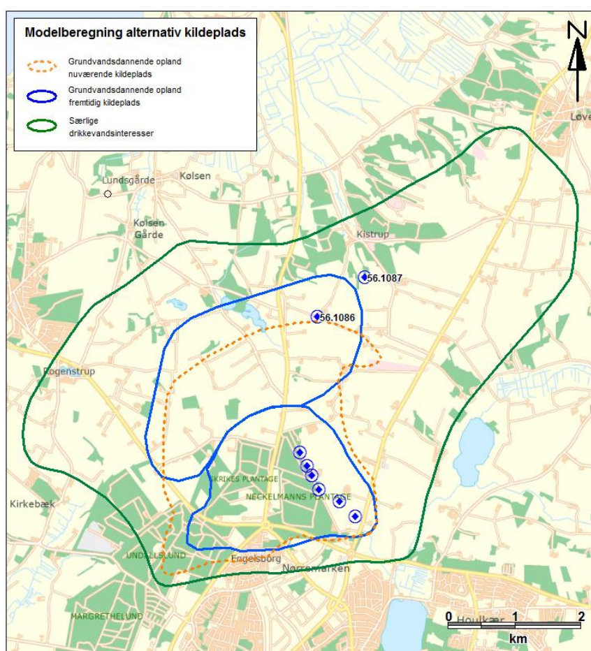
Figur 20: Modelberegning af grundvandsdannende opland hvor indvindingen til Energi Viborg Vand fordeles med 50 % på de nuværende borer og 50 % på en ny kildeplads centralt i OSD (boringerne 56.1086 og 56.1087).
