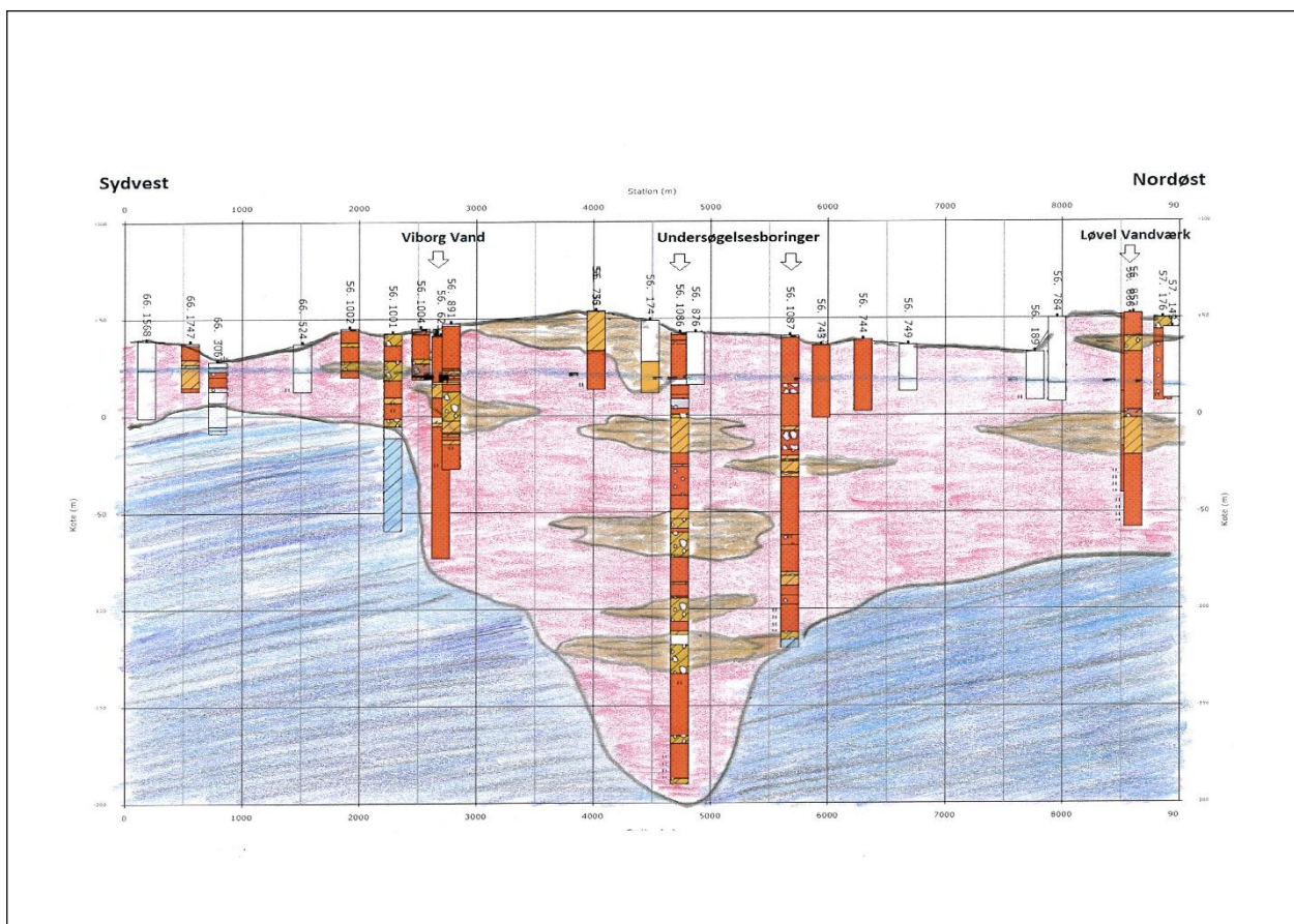
Figur 3: Skitse: Geologisk tværsnit gennem OSD Viborg Nord. Blå farver: Lag fra før istiderne, ler – finsand, dårligt eller ikke grundvandsførende. Brun farve: Smeltevandssler/moræner fra istiderne, ikke vandførende. Røde farver: Sand – grus fra istiderne, vandførende. Grundvandsspejl vist med blå linje, ca. 25 m. over havniveau. Snittets placering er vist på figur 4. Figur udarbejdet af Viborg Kommune, natur & vand.
