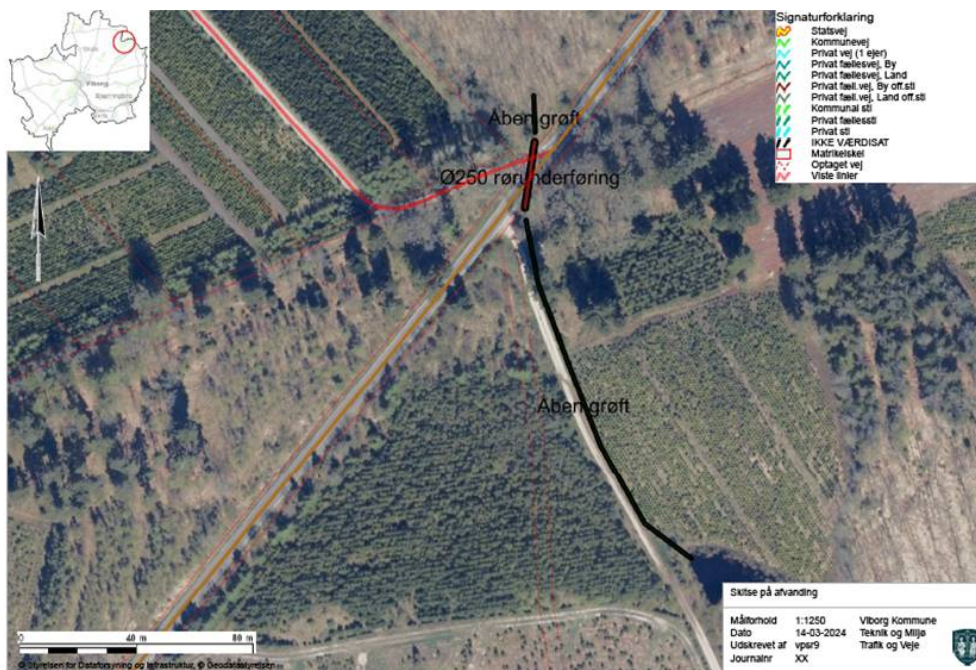
Figur 3: Trafik og Veje har aftale med lodsejer opstrøms og nedstrøms om at strømningsvejen reguleres med åbne grøfter jf. skitse.
