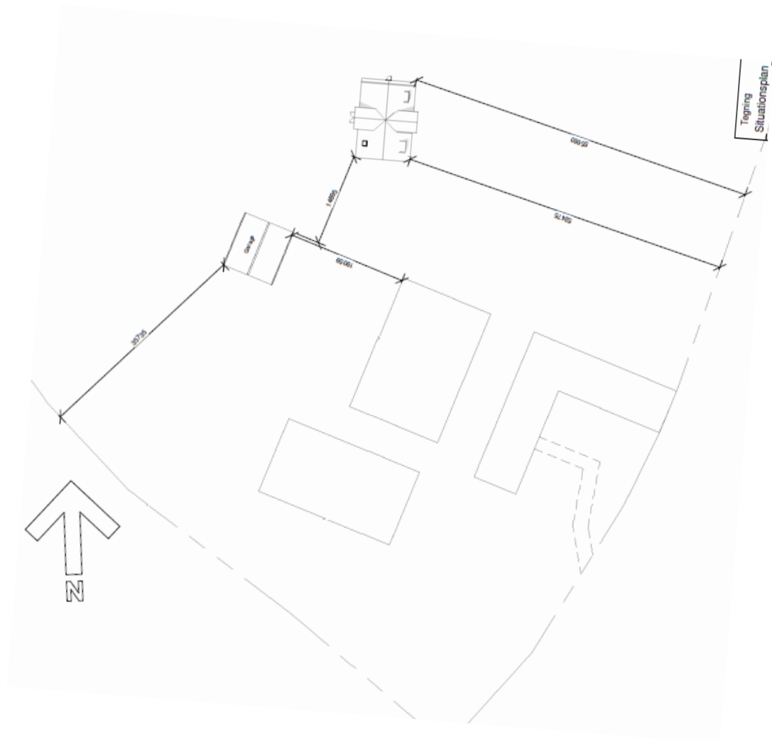
Ansøgningens situationsplan.
