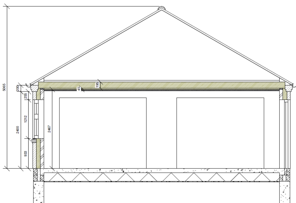
Ansøgningens snit.
