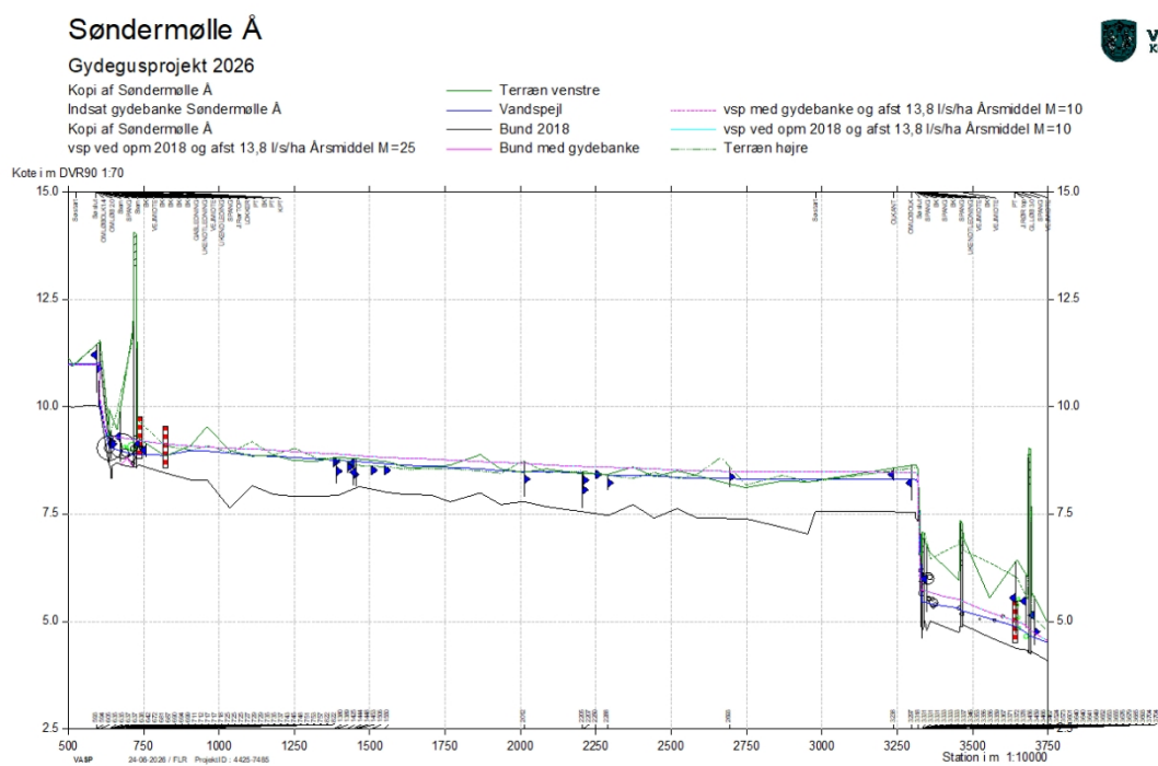
Figur 2: Længdeprofil fra VASP der viser faldforholdene mellem de to møller.
