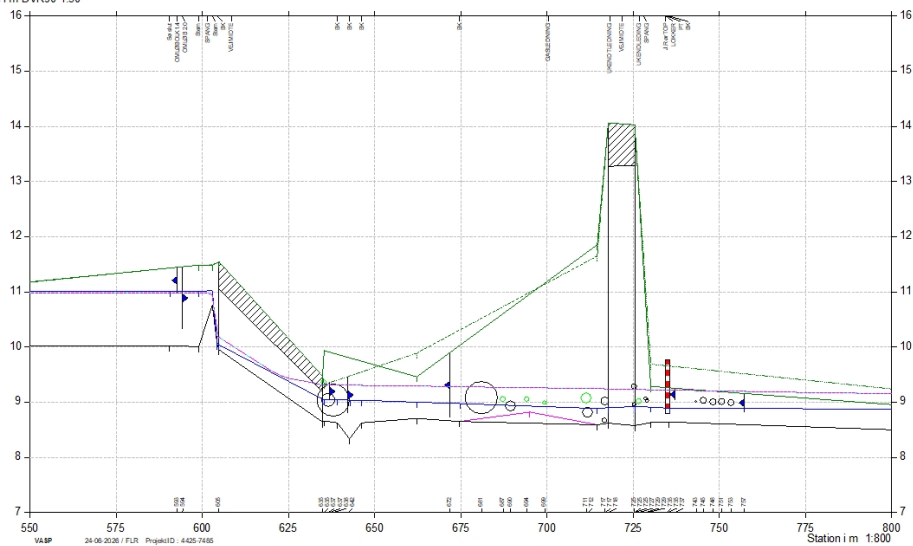
Figur 3: Længdeprofil der viser beregnede vandspejle for projektområdet.
