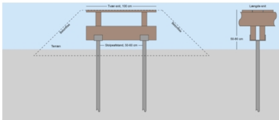
Visualisering af træstieme – der monteres dog blindekant langs begge kanter.
