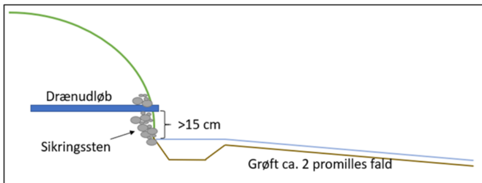
Figur 2: Skitse af etablering af drænuddløb fra ansøgningsmateriale.
