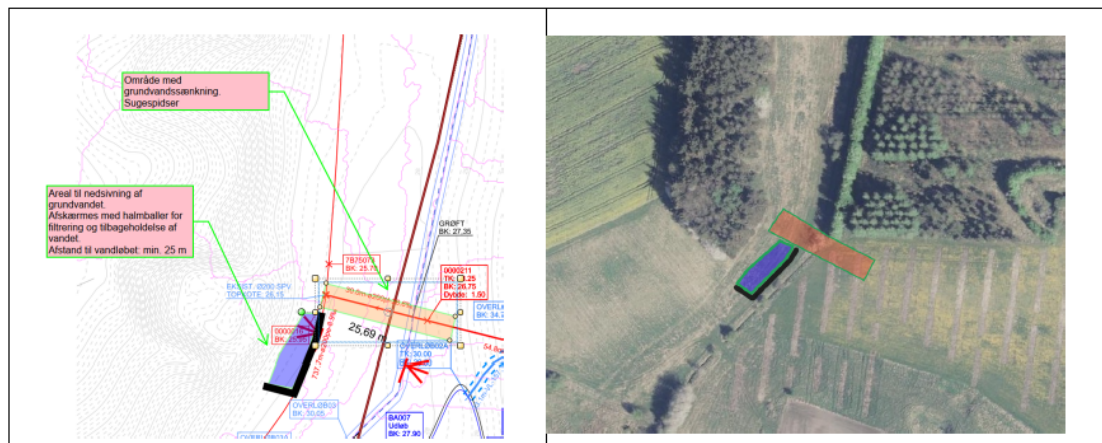
Figur 1: Placering af grundvandssænkning og areal for nedsivning. Til venstre ses placeringen fra detailplanlægningen. Til højre ses ca. placeringen på orthofoto. Orange felt angiver område for grundvandssænkning, blåt felt angiver området for nedsivning og sort linje angiver afskærmning med halmballer.
